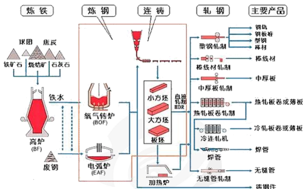
图 B.1 钢铁生产主工序
