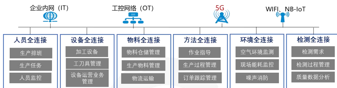
图 6 5G 全连接工厂人、机、料、法、环、测等联网内容示例
