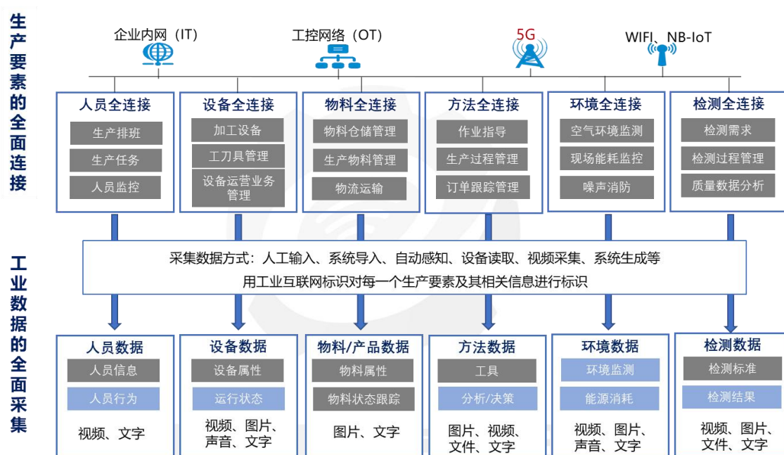
图 7 5G 全连接工厂人、机、料、法、环、测等数据采集内容示例
