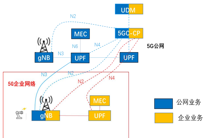
图 3 5G 混合专网部署方式
