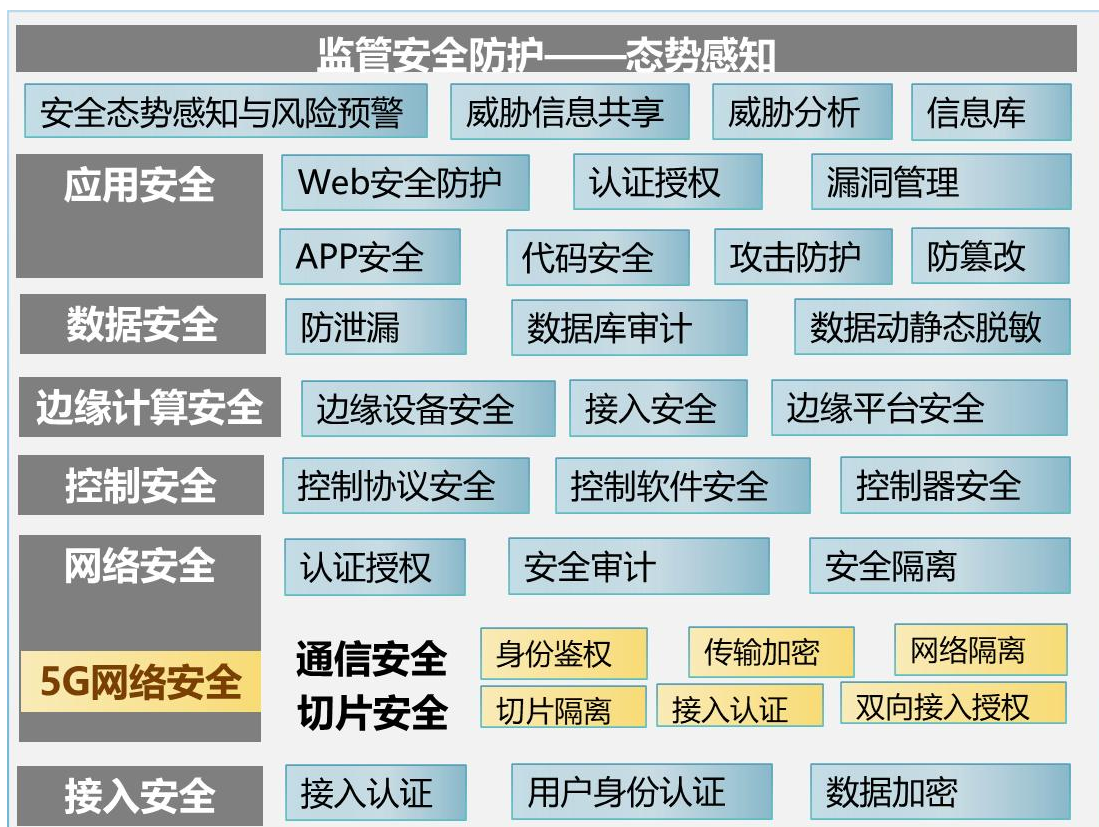
图 9 5G 全连接工厂网络安全技术体系建设
