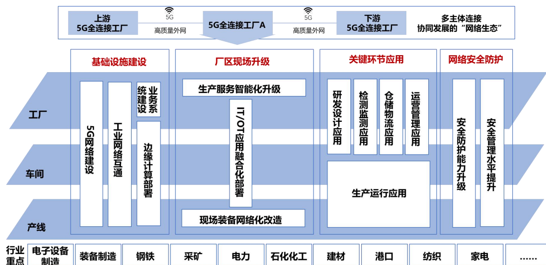
图 1 5G 全连接工厂建设框架
