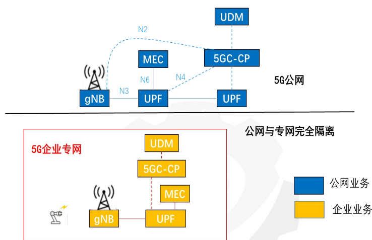
图 5 5G 独立专网部署方式
