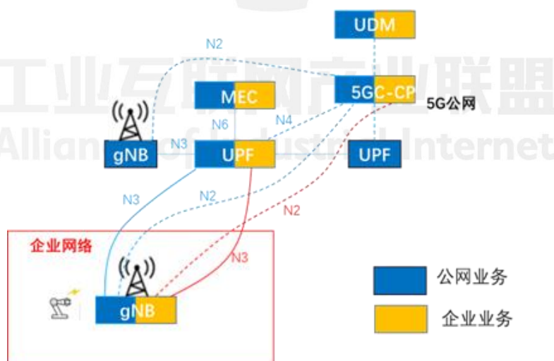
图 4 5G 虚拟专网部署方式
